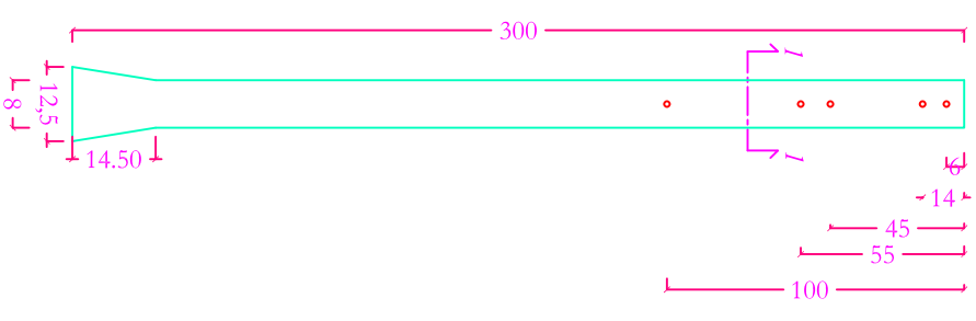
VISTA LATERALE
